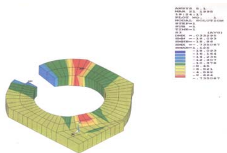
CC.1.1 PESO PROPRIO -- Tensione, DETERM. MINIMA (Q.2.2.8.3)
