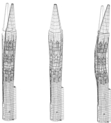
Analisi Modale
