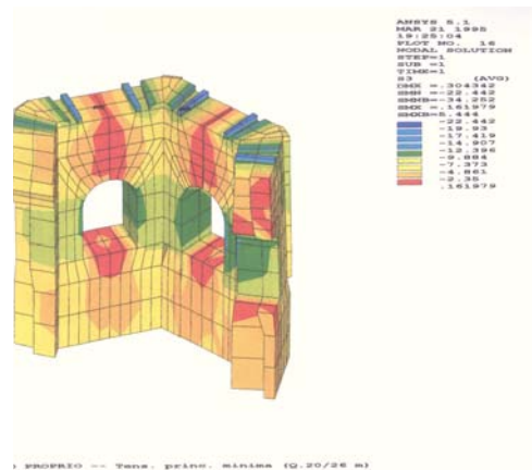
PROPRIO -- Tensione, DETERM. MINIMA (Q.20/26.3)
